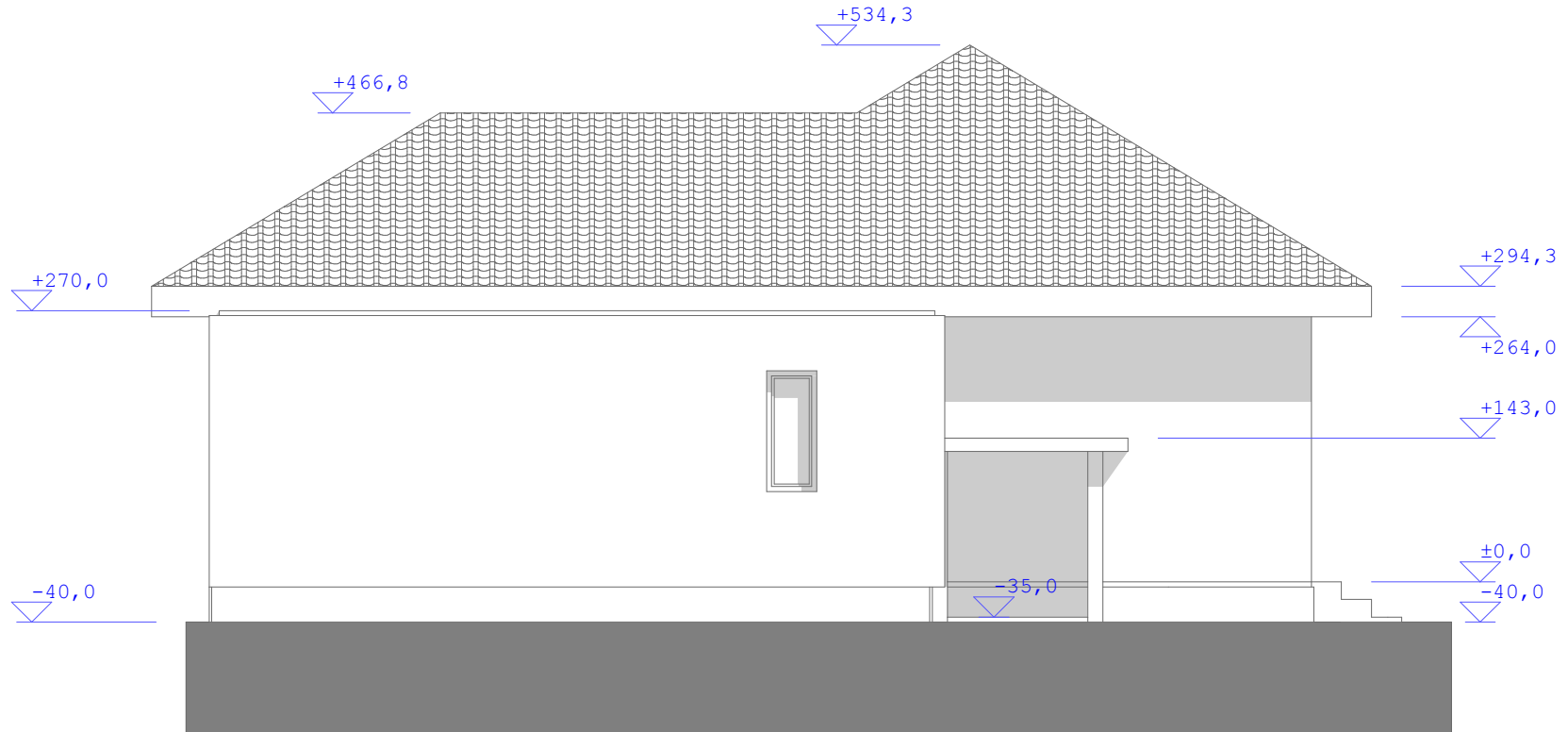
FATADA NORD-VEST - SITUATIA EXISTENTA 1:70
